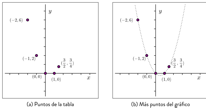
Figura 4.1: Gráfico de la función f
