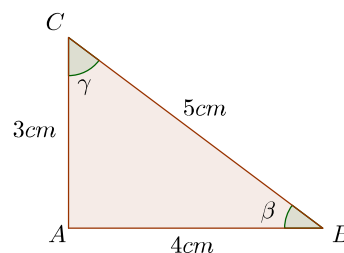
Figura 5.29: Triángulo del Ejemplo ??
