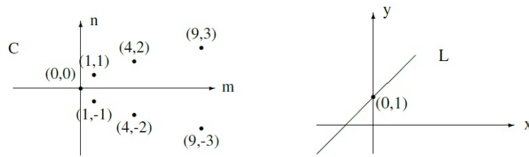
Figura 3.16: Representación gráfica de los conjuntos C y L
