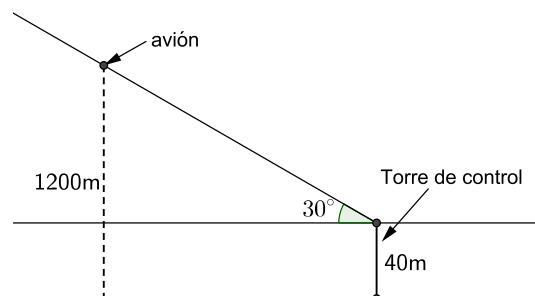
Figura 5.34: Esquema del ejercicio ??
