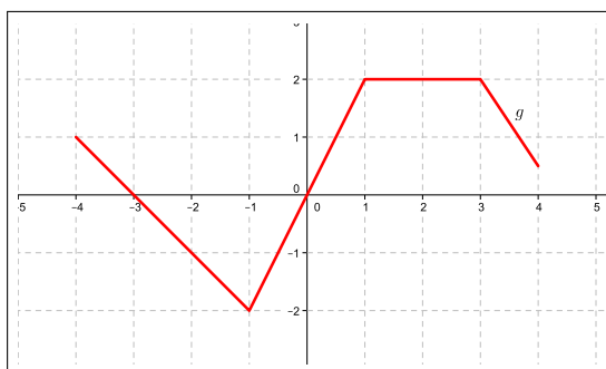
Figura 4.39: (Ejercicio ??)-Gráfico de g .
