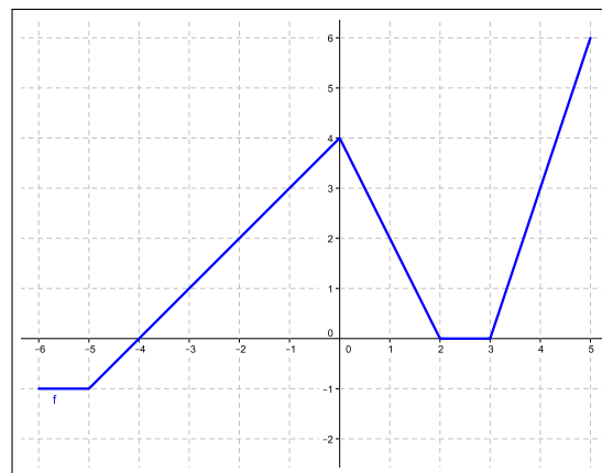
Figura 4.38: (Ejercicio ??)-Gráfico de f .
