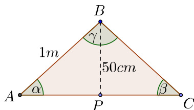
Figura 5.31: Triángulo del Ejemplo ??
