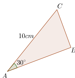
Figura 5.30: Triángulo del Ejemplo ??
