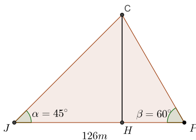
Figura 5.32: Triángulo del Ejemplo ??
