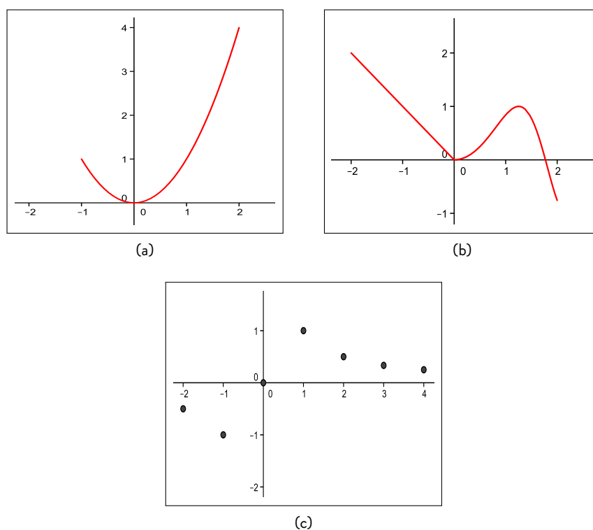
Figura 4.2: Gráficos de funciones
